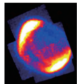
超新星残骸SN1006のX線像(あすか衛星撮影：JAXA提供)
