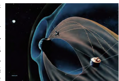
地球磁気圏と探査衛星
